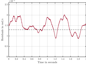
(d) Fault group 2 - Severity level 1 (F2/SV1) residuals
